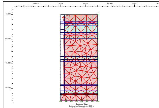
Simulation von Bruchvorgängen (FEM)
