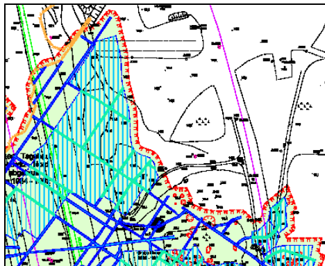
Auszug Betriebsrisswerk Grube Elvira, Lichterfeld
