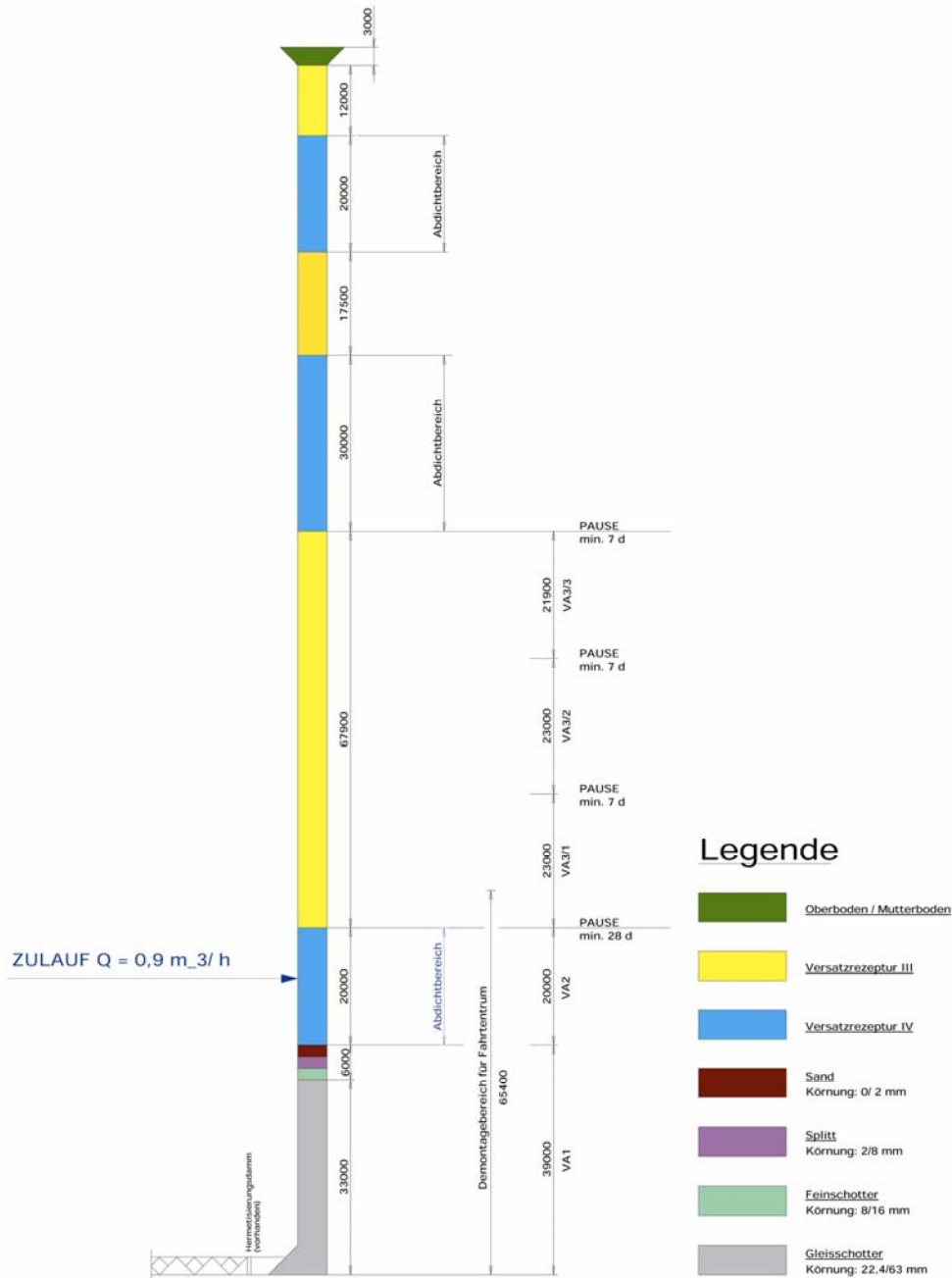
Darstellung der Füllsäule am Beispiel des Schachtes 392 (Grundsohle und Schacht nicht befahrbar)
