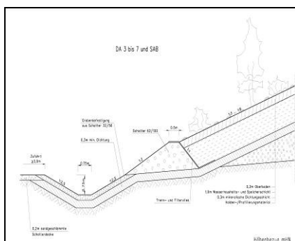
Bild: Ausbildung Böschungsfuß
