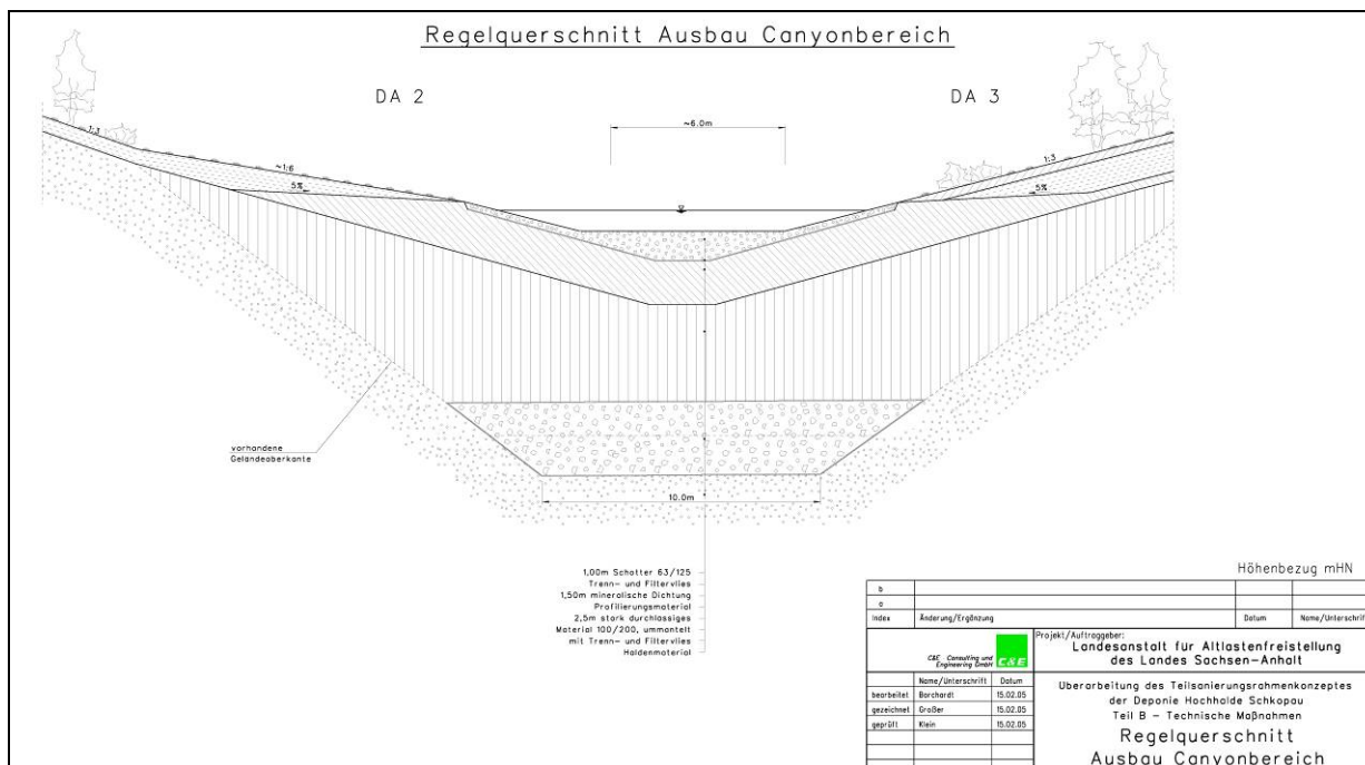
Bild: Regelquerschnitt Ausbau des alten Lauchabettes
