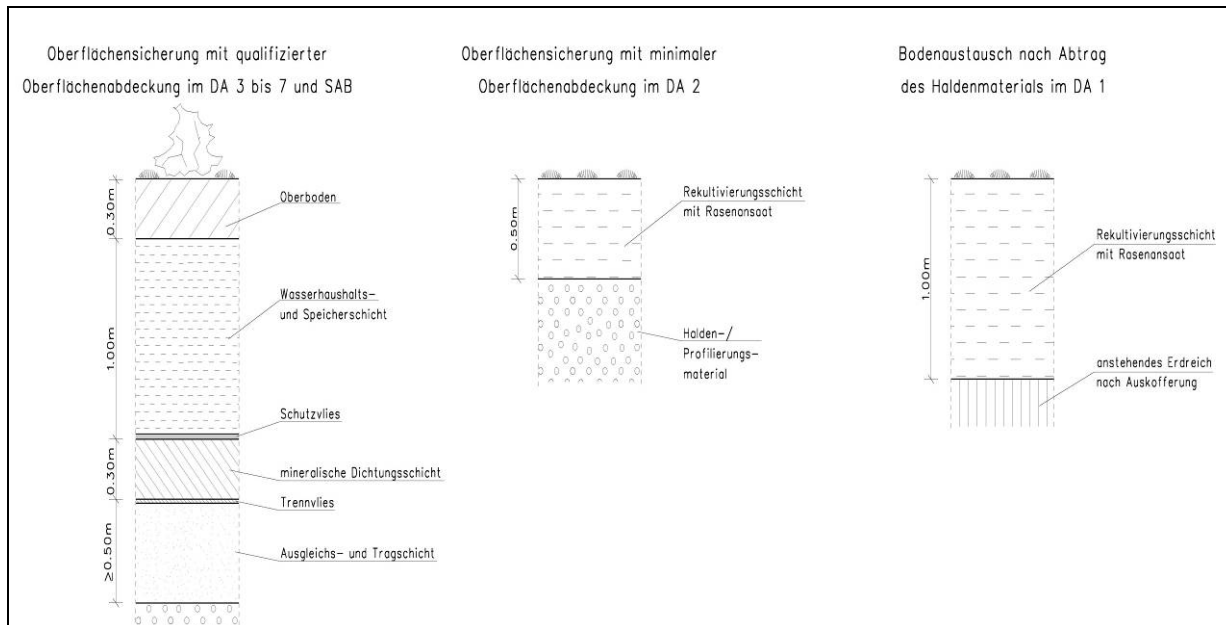
Bild: Regelaufbau der Oberflächensicherungssysteme
