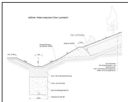
Bild: südlicher Haldenrandgraben
